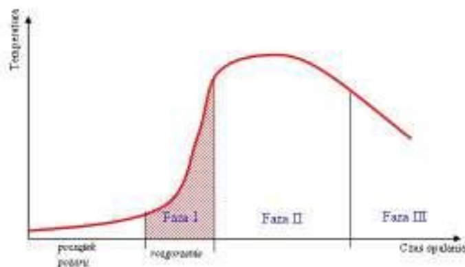
Wykres 1. Fazy rozwoju pożaru wewnętrznego
